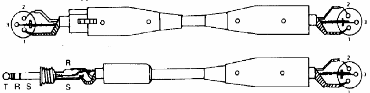
Рис.1 Микрофонные входы (XLR-3)
