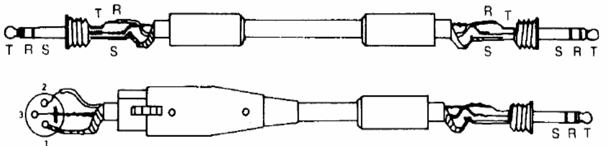
Рис. 1-2 Линейный вход
