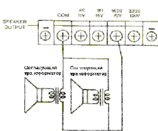
Подключение нагрузки 16Ω
