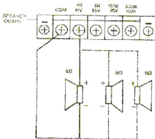
Подключение нагрузки 4 ома
