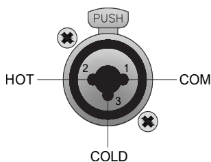
Входной комбинированный разъем
