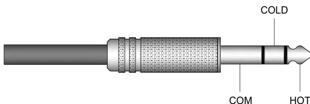
Штекер Jack 6.3
