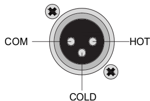
Штекер XLR
